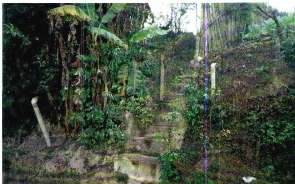
Foto 26 - Rede de esgoto passando em terrenos particulares, de forma elevada sobre o solo. Deverão ser adaptadas em parte
